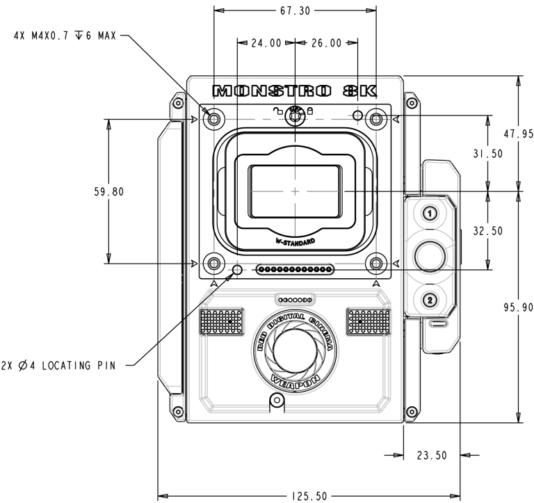
Figure: 具备 MONSTRO 8K VV 传感器的 WEAPON 正面视图
