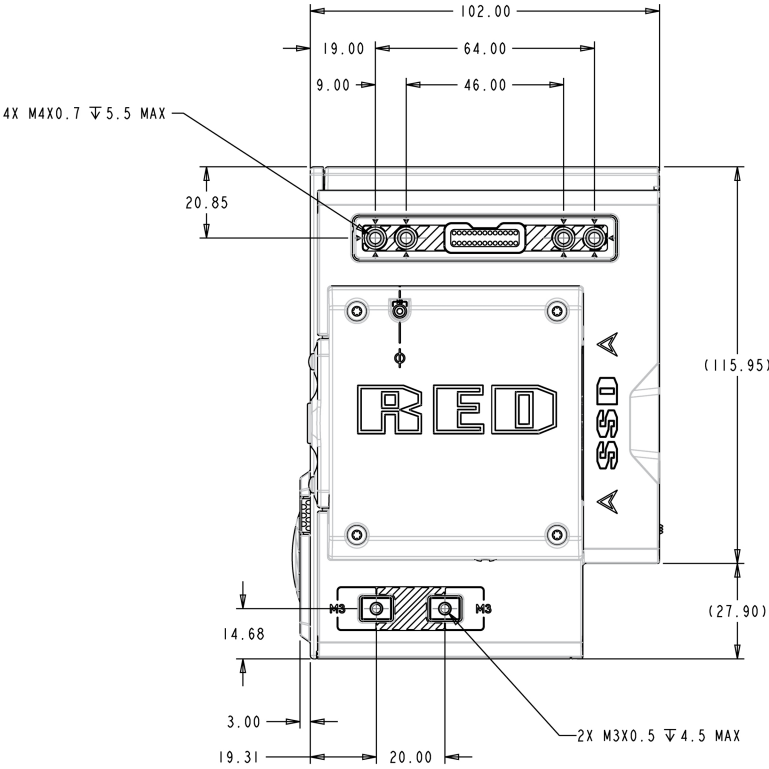
Figure: 具备 MONSTRO 8K VV 传感器的 WEAPON侧面视图( 右侧)
