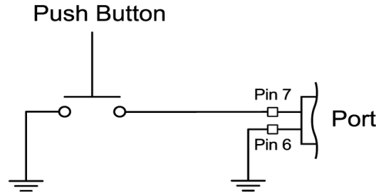
Figure: 触点闭合式触发器按钮电路图 (SYNC)
