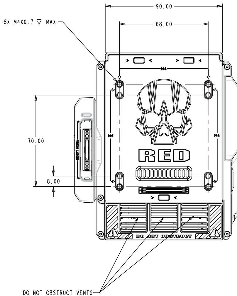
Figure: 具备 MONSTRO 8K VV 传感器的 WEAPON 背面视图
