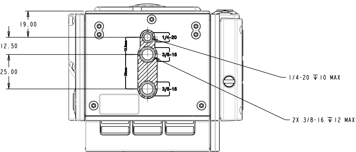
Figure: 具备 MONSTRO 8K VV 传感器的 WEAPON底部视图
