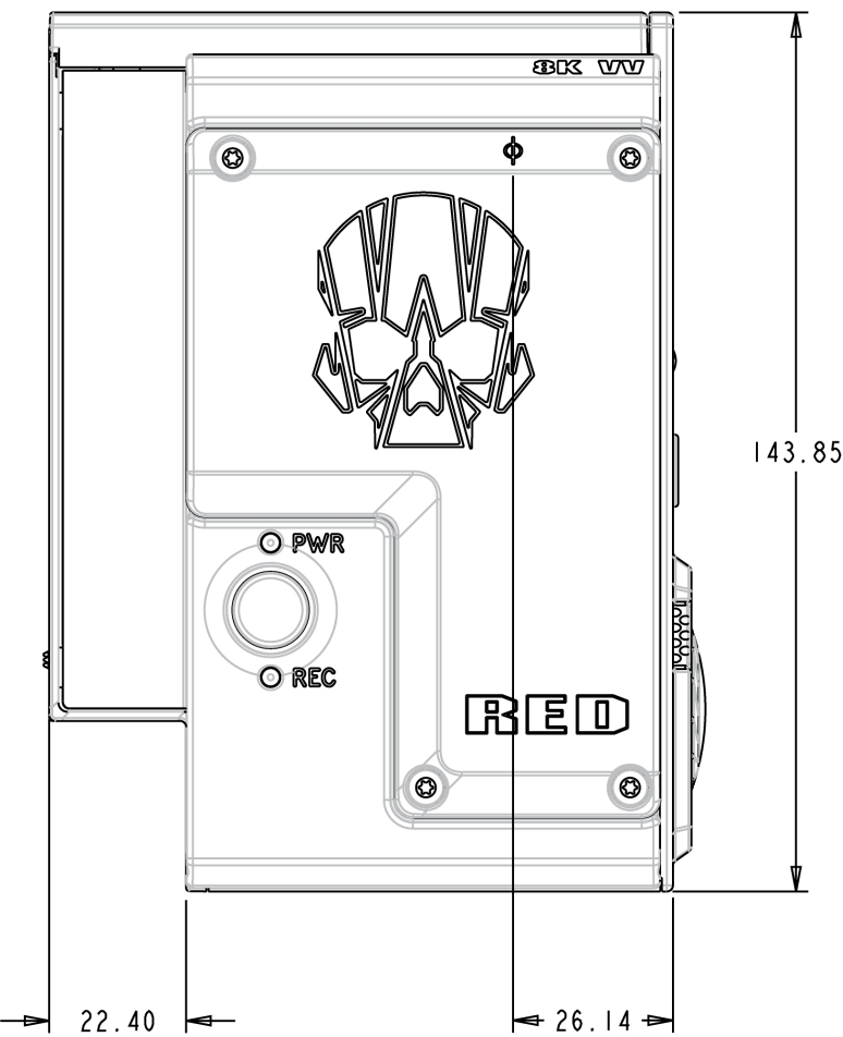
侧面视图( 左侧)
