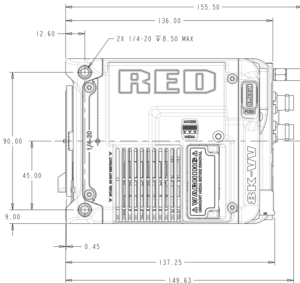
图。相机侧视图(左)
