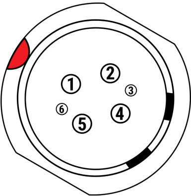
图。雄性6针1L直流电源输入连接器的正面( 看着相机的背面) 。
