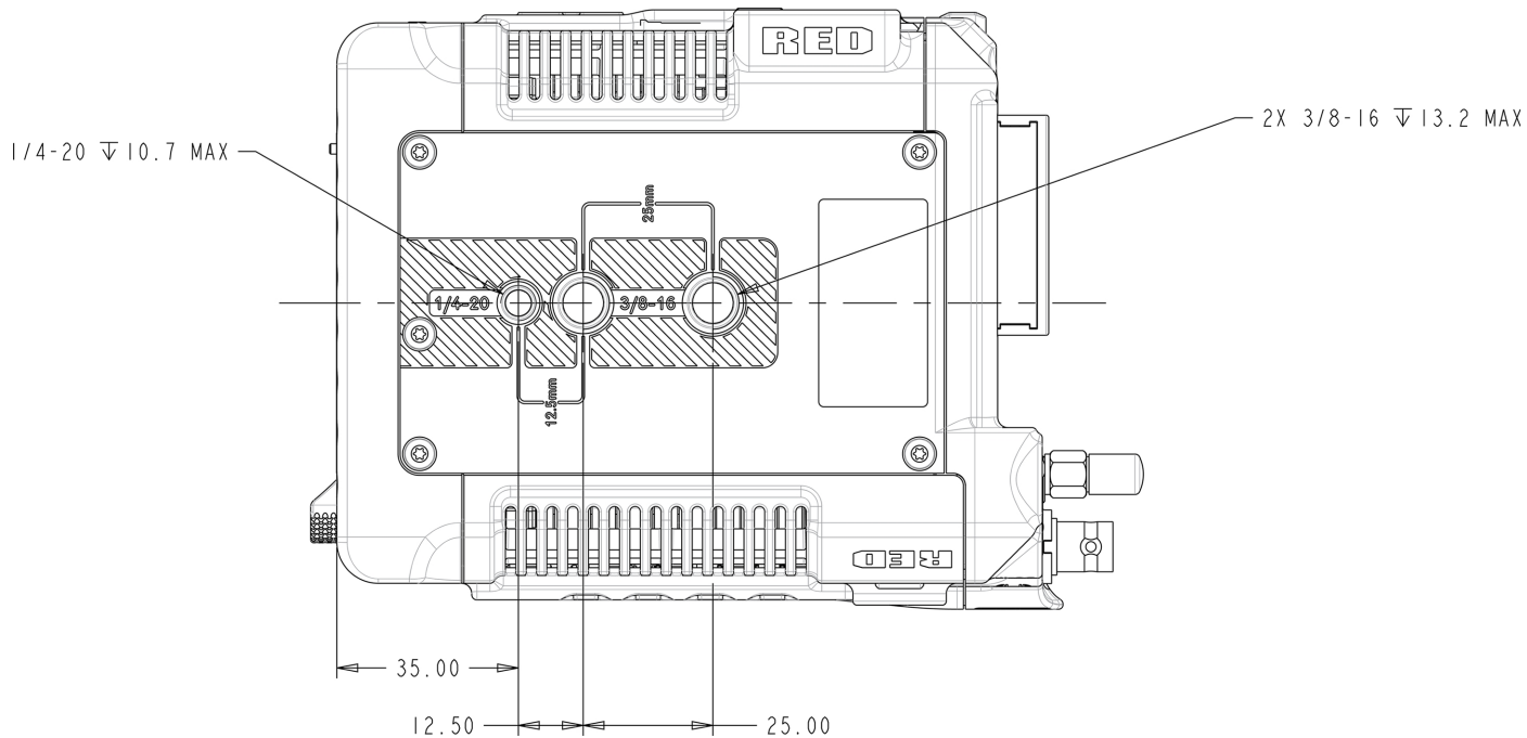
图。摄像机底视图
