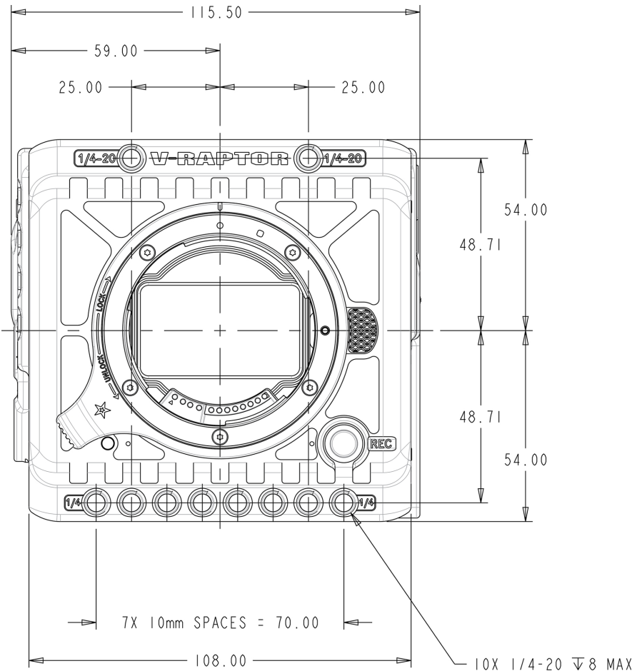
图。摄像机前视图
