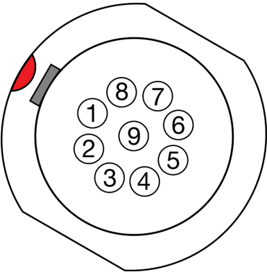
图. 雌性9触点扩展端口的正面( 看着相机的背面) 。
