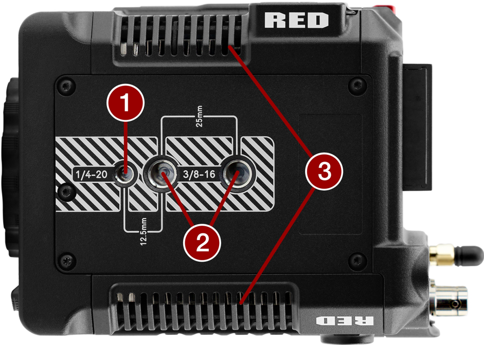
图。相机机身底部特征
