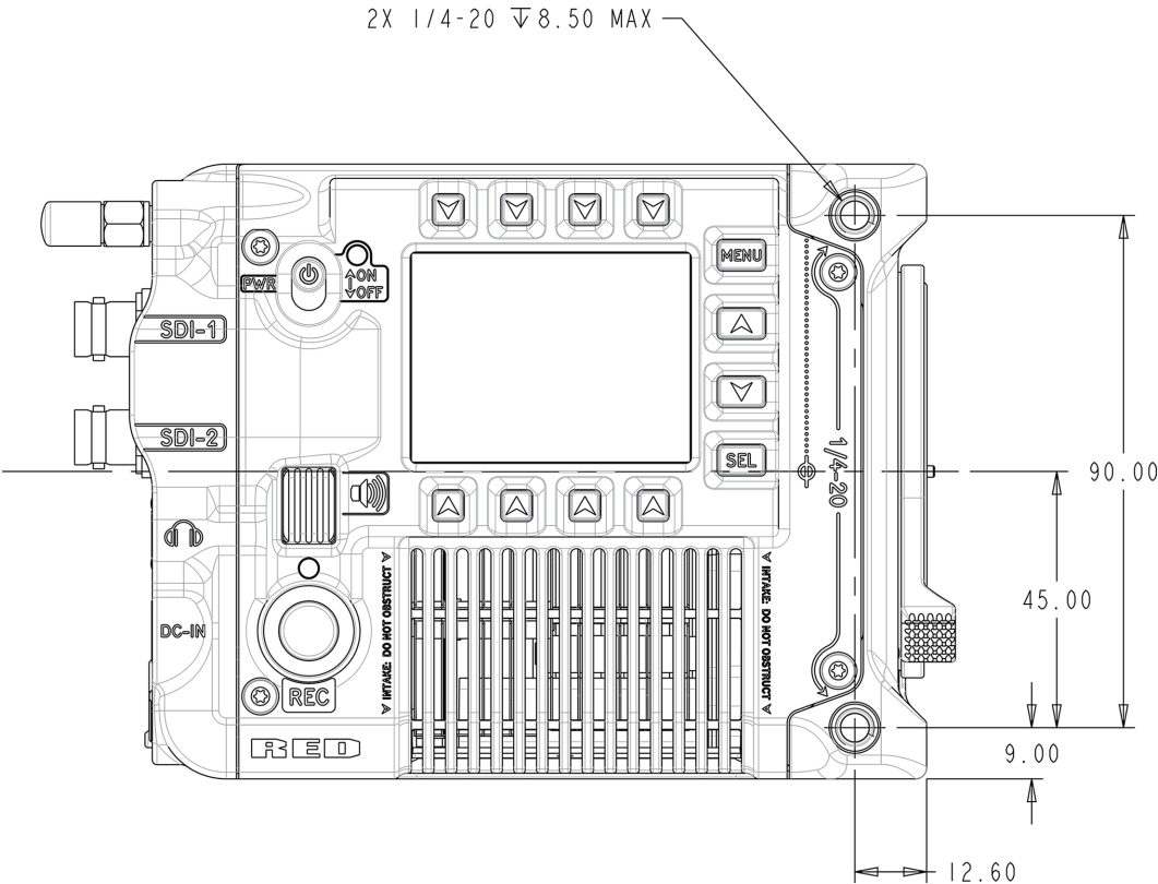
图。相机侧视图(右)。
