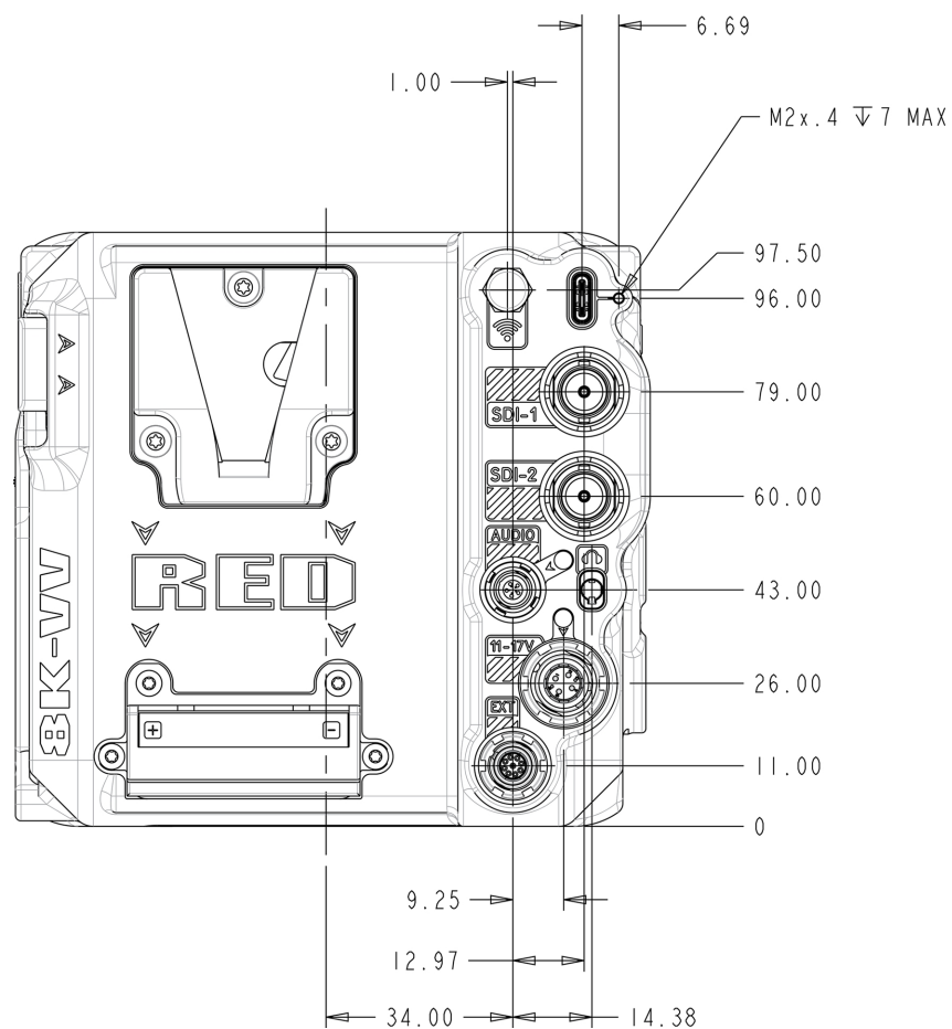
图。摄像机后视图(V型锁)
