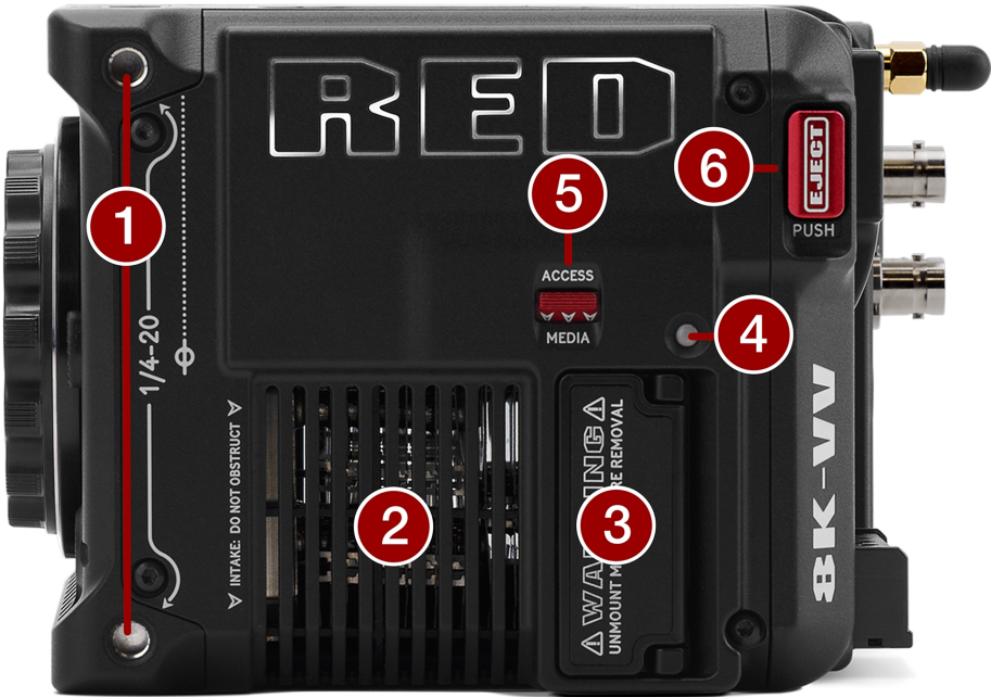
图。相机机身左侧控制和功能
