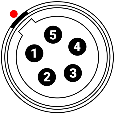
图。雌性5针00B音频连接器的正面( 看着相机的背面) 。
