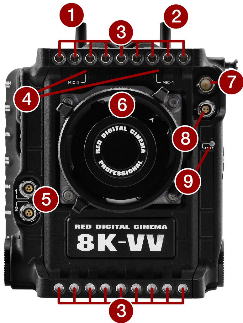
Figure: 相机机身正面，控制和功能
