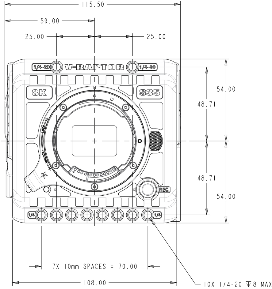
Figure: 摄像机前视图
