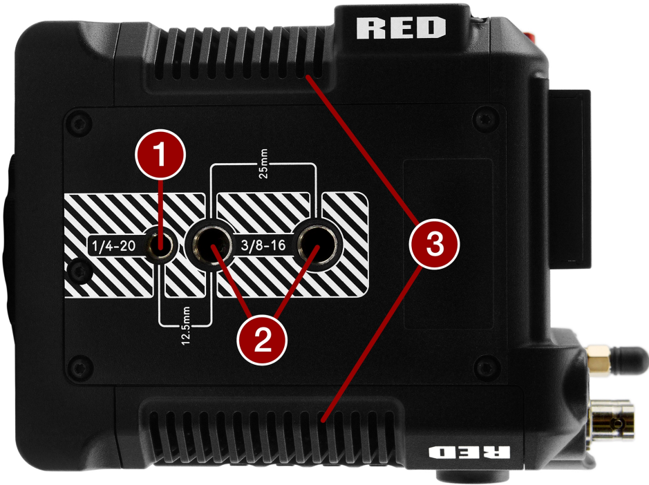
Figura: Características inferiores del cuerpo de la cámara
