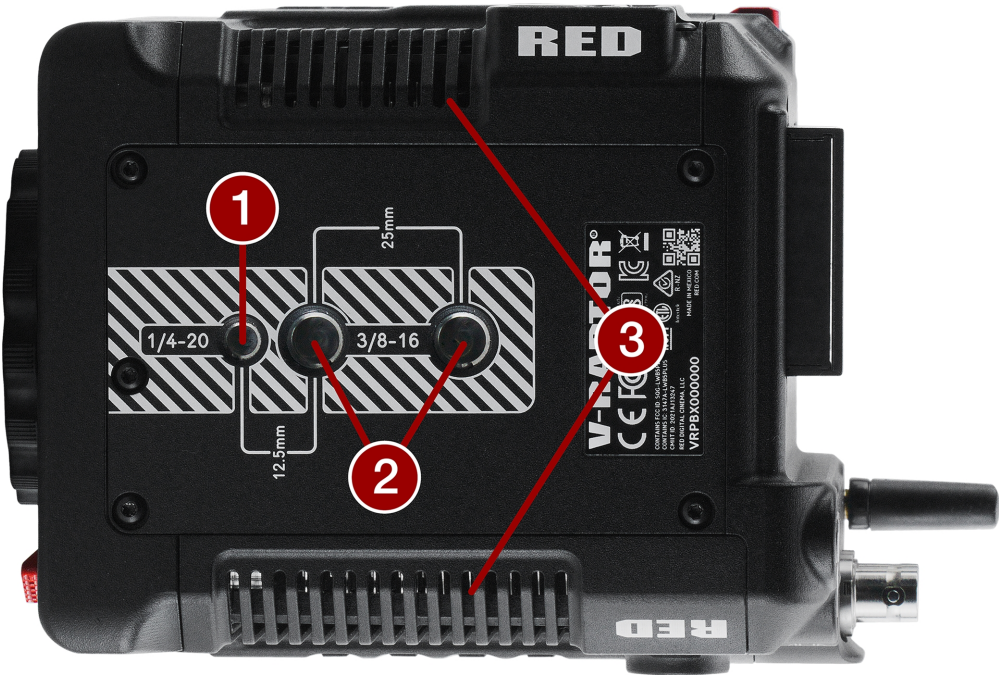
Figure: 相机机身底部特征
