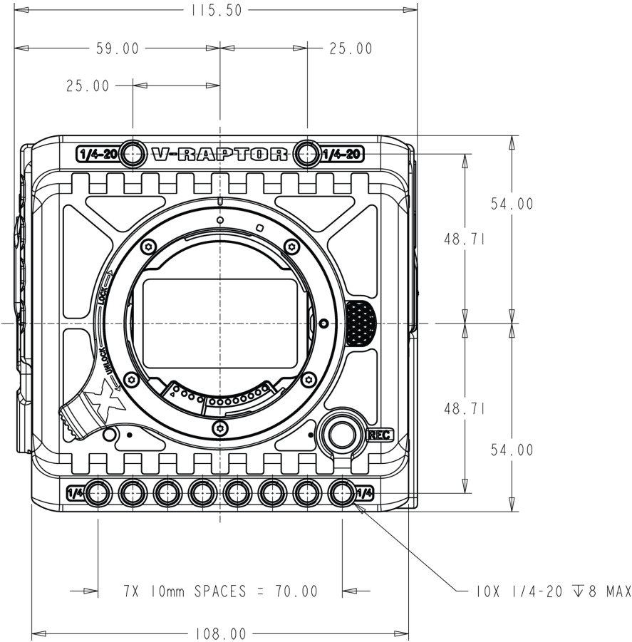
Figure: 摄像机前视图
