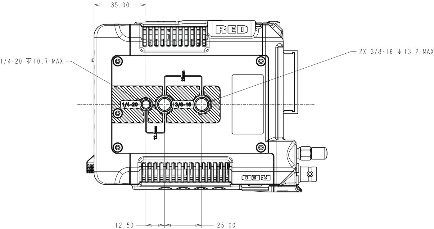
Figura: Vista inferior de la cámara
