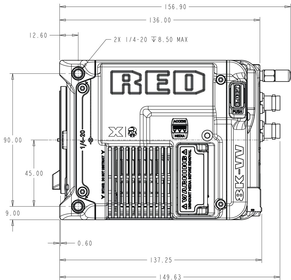
Figura: Vista lateral de la cámara (izquierda)
