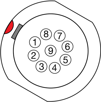
Figura: Cara frontal de extensión hembra de 9 contactos (mirando hacia la parte posterior de la cámara).
