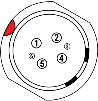
Figura: Cara frontal del conector macho de 6 patillas 1B de entrada de corriente continua (mirando hacia la parte posterior de la cámara).
