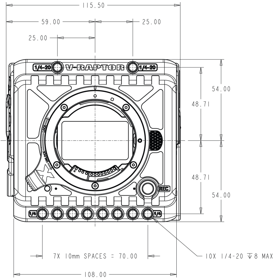
Figure : Caméra vue de face
