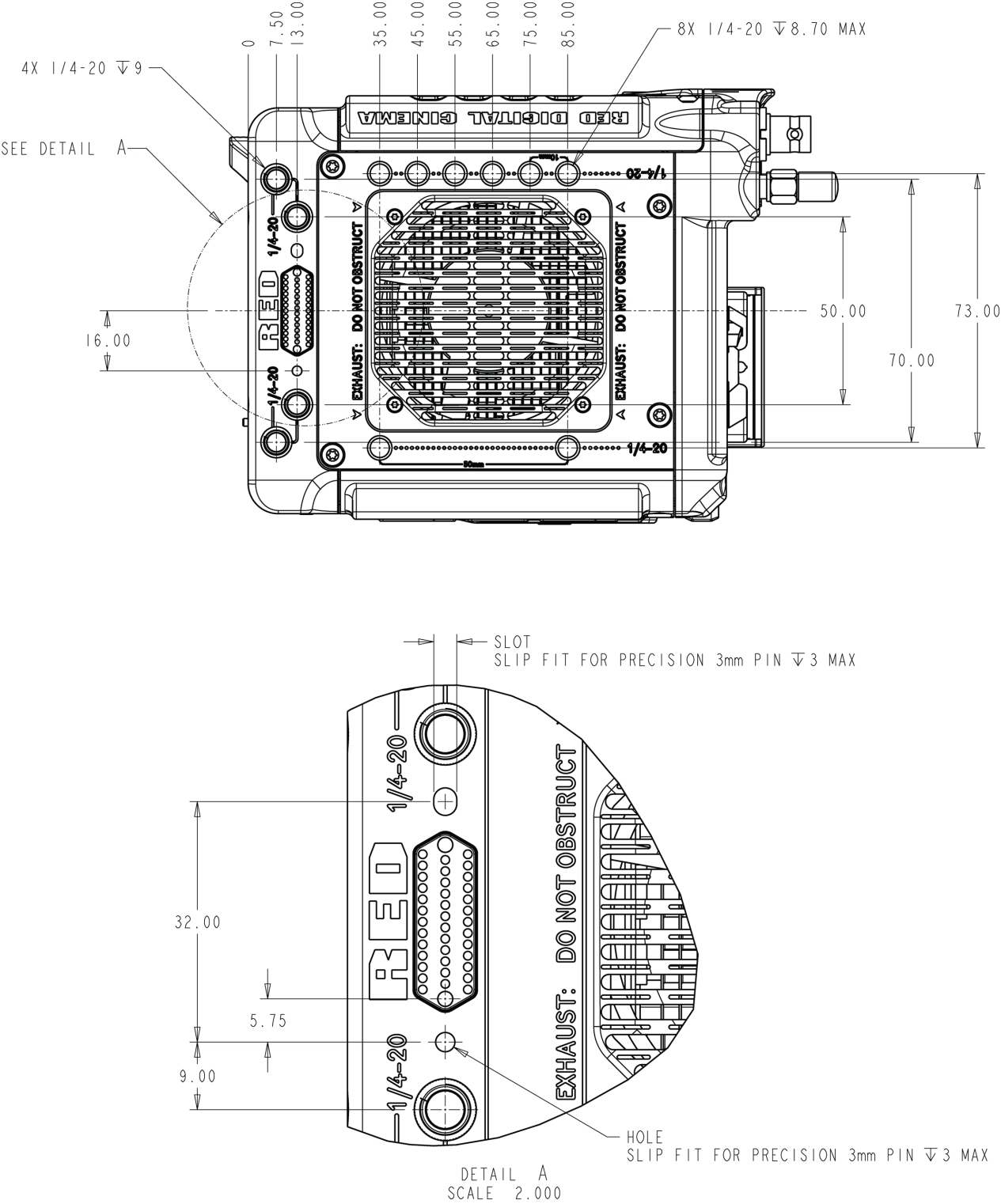
Figure : Vue de dessus de la caméra
