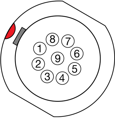
Figure : Face avant du port d'extension femelle à 9 contacts (en regardant l'arrière de la caméra). NOTE : Le connecteur correspondant requis est le connecteur droit à 9-pin 0L (ODU, part# SX0L0X-P09MCC0-0001).
