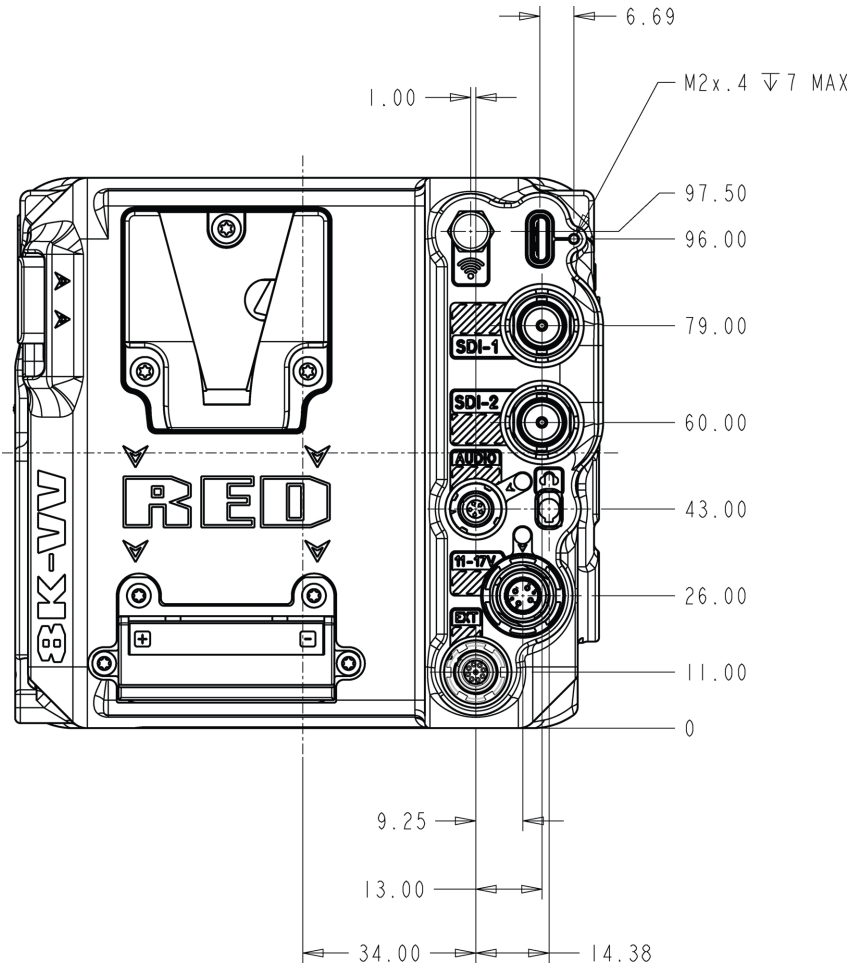
Figure : Vue arrière de la caméra
