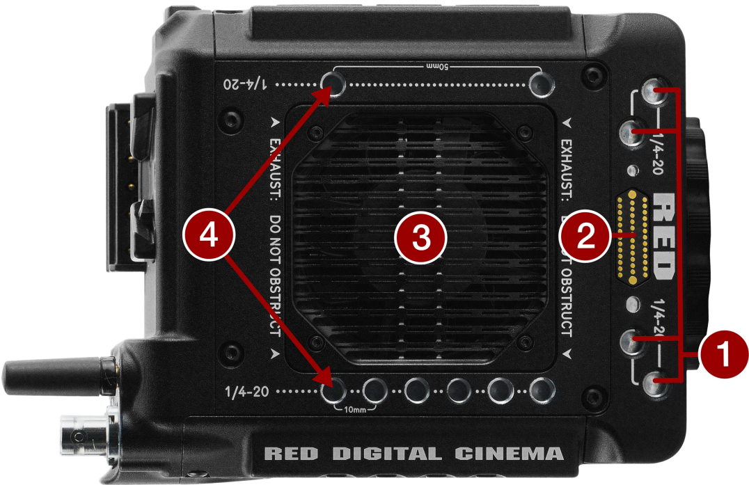
Figure : Commandes et fonctions supérieures du boîtier de la caméra
