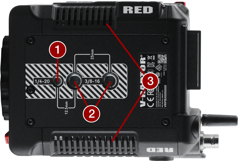
Figure : Caractéristiques du fond du boîtier dela caméra
