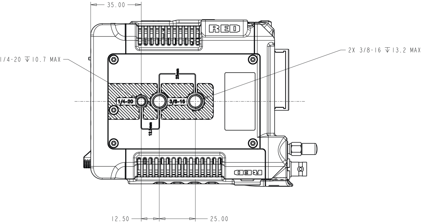
Figure : Vue du dessous de la caméra
