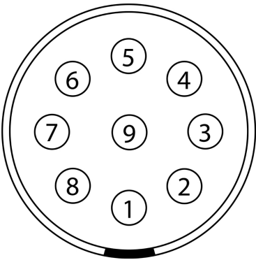
Figure :GIG-E连接器的正面( 看着相机的背面) 。
