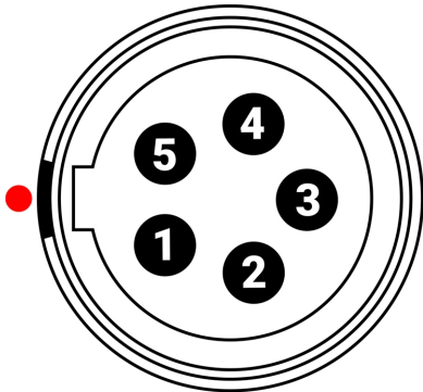
Figure : 雌性5针00B 音频连接器的正面( 看着相机的背面) 。
