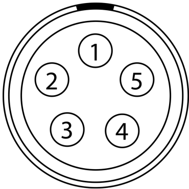
Figure : 时间码 0B 连接器的正面( 看着摄像机的背面) 。
