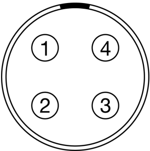
Figure : 雌性4针00B CTRL连接器的正面( 看着摄像机的背面) 。
