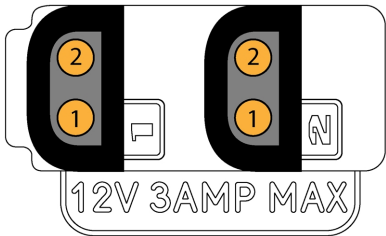
Figure: 无盖 P-Tap 连接器的正面( 从相机顶部看) 。
