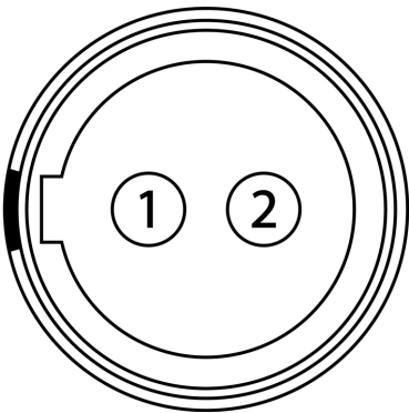
Figure :2针AUX EVF母接头的正面( 看着相机的正面) 。
