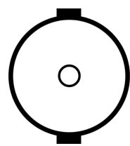
Figure :Genlock公头BNC连接器的正面( 看着摄像机的背面) 。
