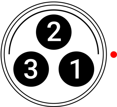
Figure: 费舍尔母接头的正面( 看着相机的正面) 。
