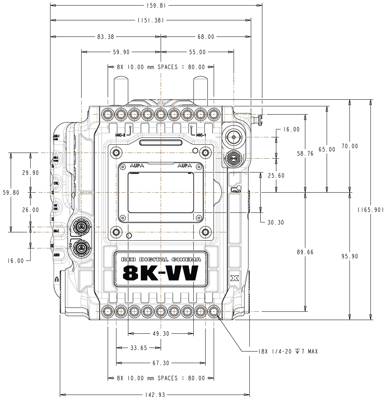
Figure: 摄像机前视图
