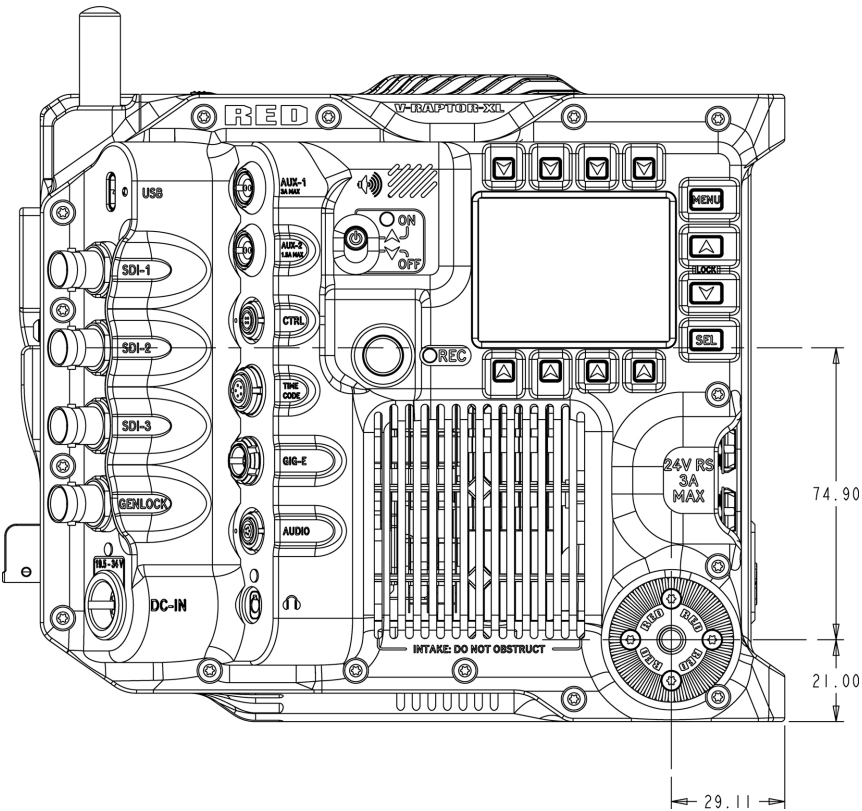
Figure : 相机侧视图( 右) 。
