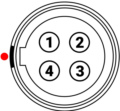
Figure : 雄性DC-IN电源输入连接器的正面( 看着相机的背面) 。
