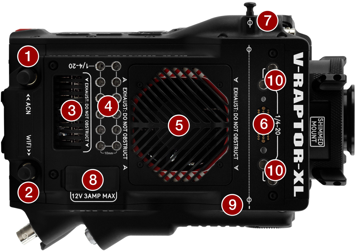
Figure：相机机身顶部、控制和功能
