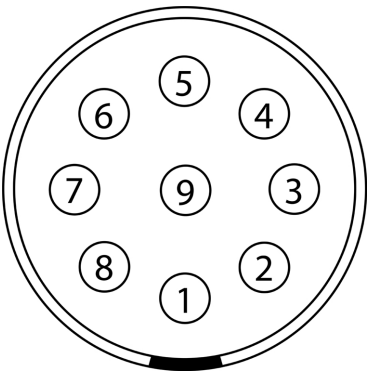
Figura: Cara frontal del conector GIG-E (mirando a la parte posterior de la cámara).
