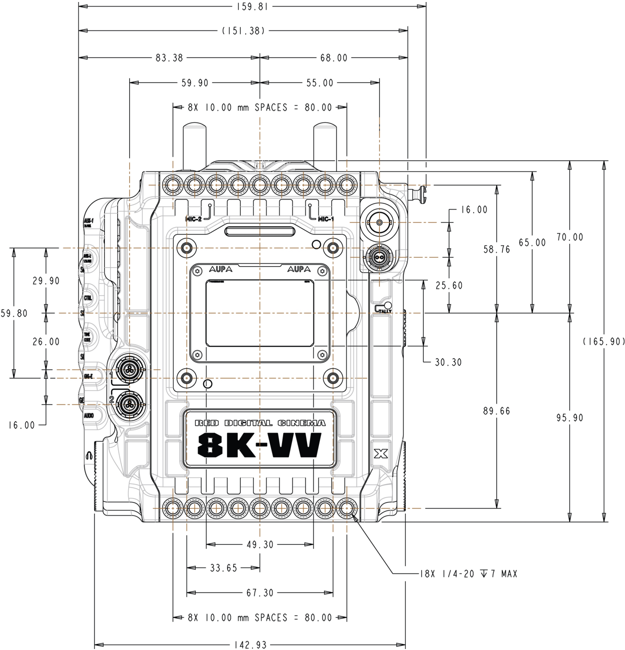
Figura: Vista frontal de la cámara
