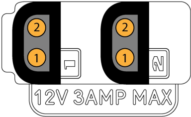
Figura: Cara frontal de los conectores P-Tap descubiertos (mirando a la parte superior de la cámara).
