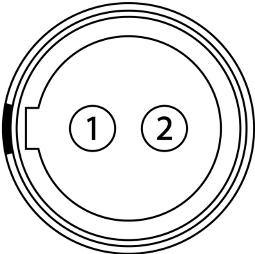
Figura: Cara frontal del conector AUX-1 hembra (mirando a la parte posterior de la cámara).
