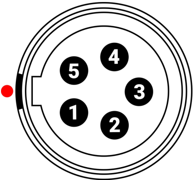
Figura: Cara frontal del conector de audio 00B hembra de 5 patillas (mirando a la parte posterior de la cámara).
