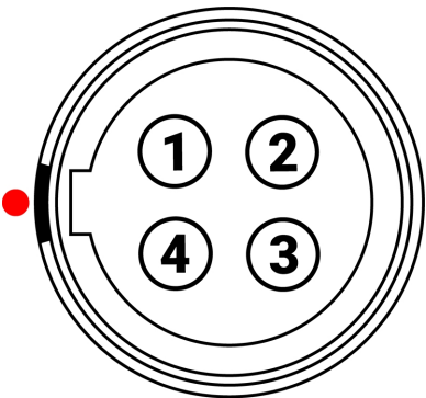
Figura: Cara frontal del conector macho de entrada de alimentación DC-IN (mirando hacia la parte posterior de la cámara).
