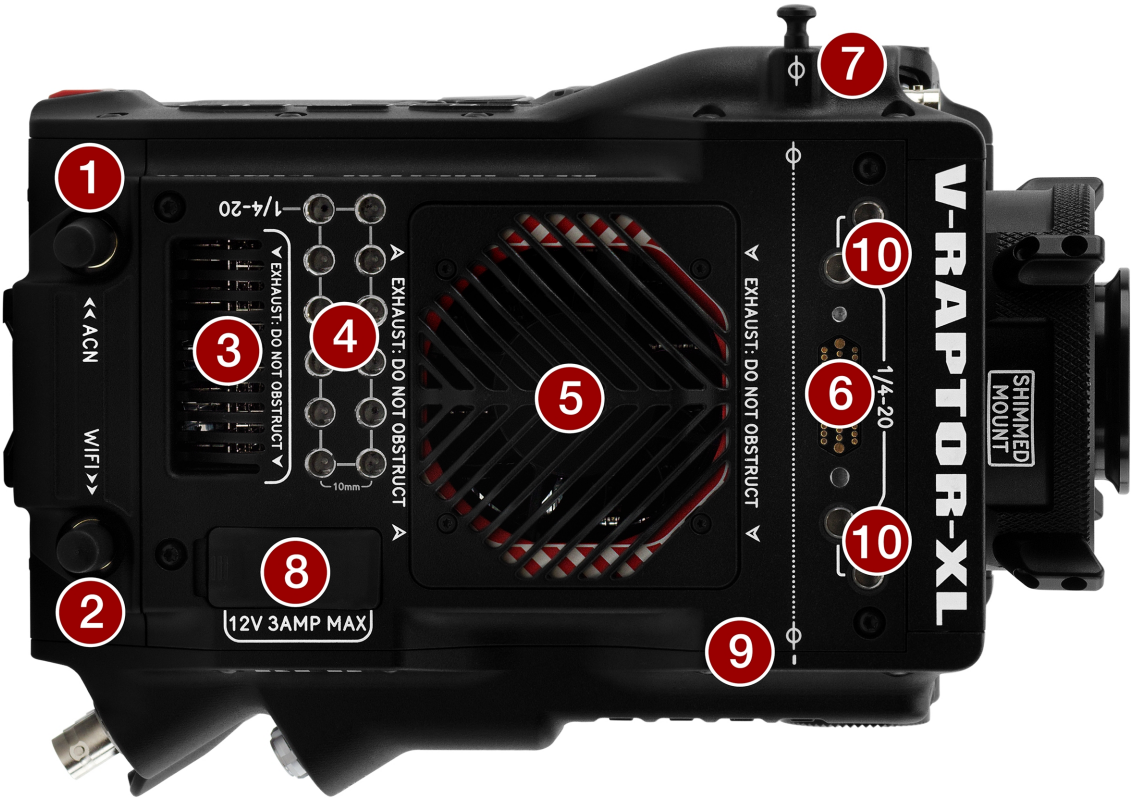
Figura: Parte superior del cuerpo de la cámara, controles y funciones
