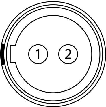
Figura: Cara frontal del conector hembra AUX EVF de 2 patillas (mirando a la parte frontal de la cámara).
