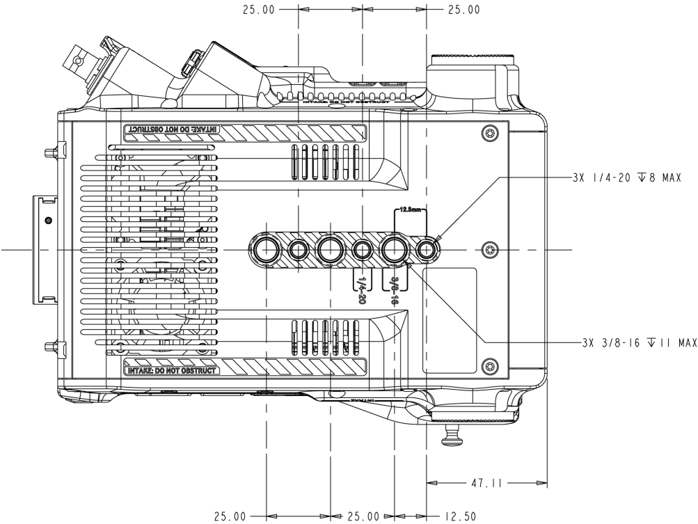
Figura: Vista inferior de la cámara
