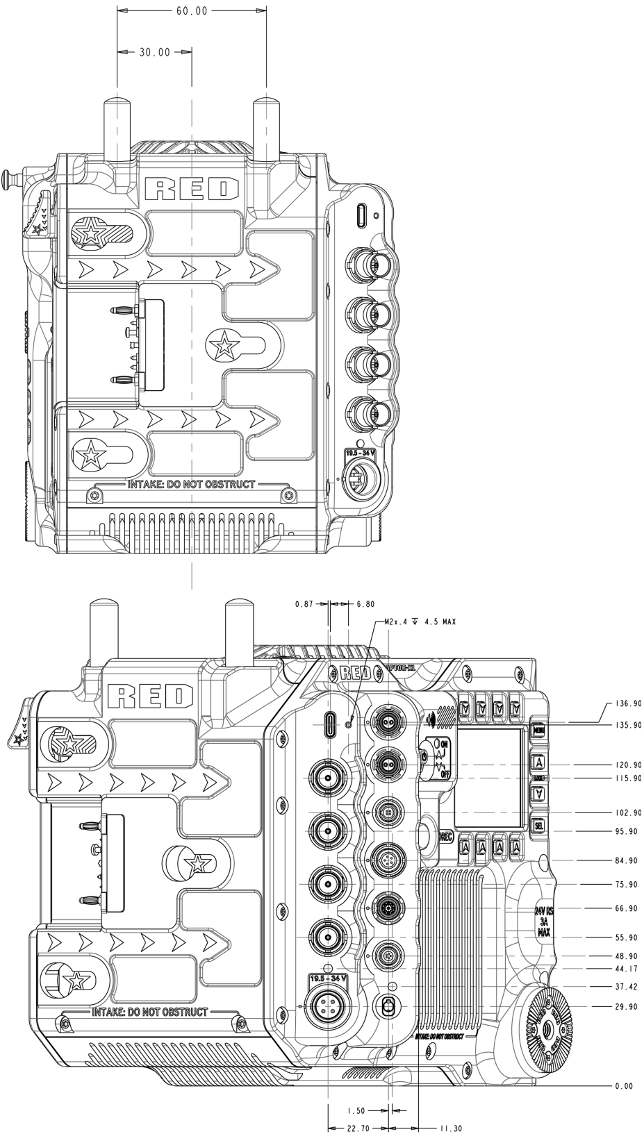
Figura: Vista trasera de la cámara (montaje dorado)
