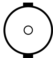
Figura: Cara frontal de los conectores BNC macho SDI 12G (mirando a la parte posterior de la cámara).
