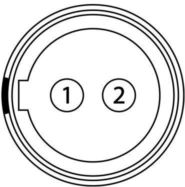
Figura: Cara frontal del conector AUX-2 hembra (mirando a la parte posterior de la cámara).
