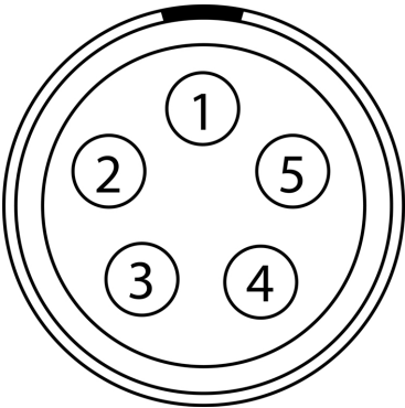
Figura: Cara frontal del conector Timecode 0B (mirando a la parte trasera de la cámara).
