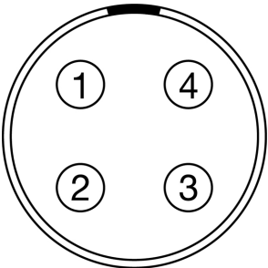
Figura: Cara frontal del conector hembra 00B CTRL de 4 patillas (mirando a la parte posterior de la cámara). El conector hembra LEMO de 4 patillas 00B CTRL admite el control remoto RS-232 para la comunicación con cámaras 3D y aplicaciones de ingesta de metadatos de terceros.
